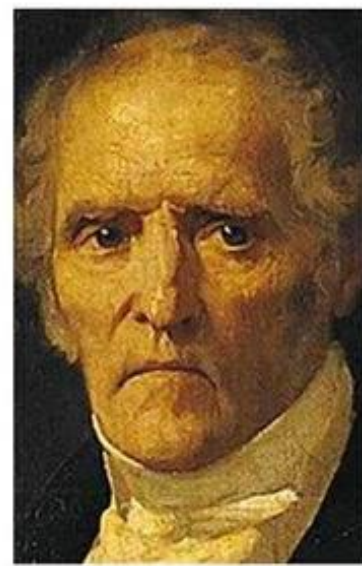
傅立叶
