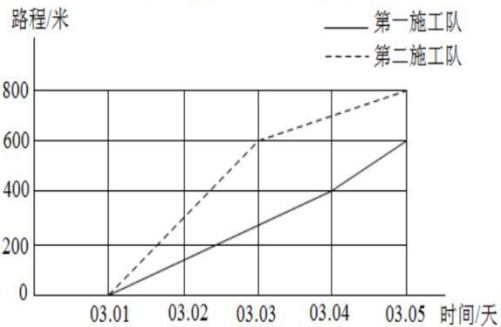
两个施工队共同修建一条水渠情况统计图
