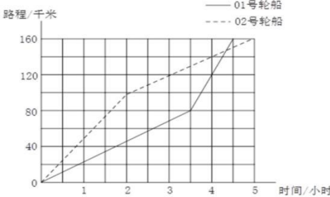
从同一港口出发的两艘轮船的运行情况统计图
