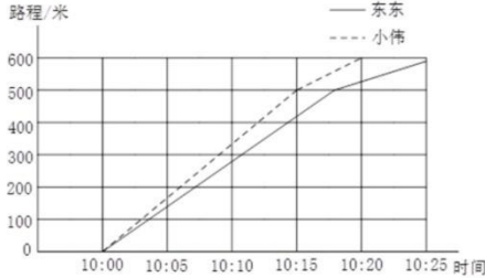
东东和小伟爬山比赛情况统计图
