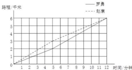
罗勇和赵康6千米骑自行车比赛情况统计图
