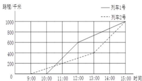
两列火车从北京到南京运行情况统计图
