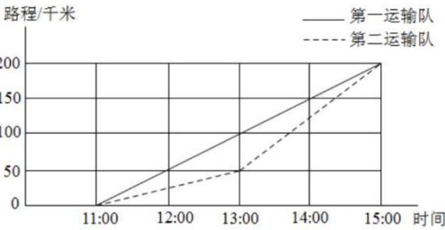
两个运输队运输粮食运途情况统计图
