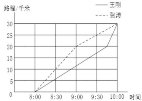
两名战士30千米越野测试情况统计图
