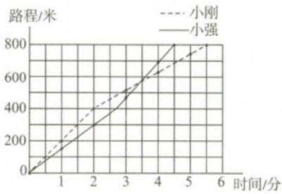
小刚和小强800米跑步情况统计图
